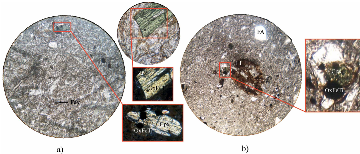
Figura 4. Secciones delgadas representativas de la Ignimbrita Toba San Felipe en Cataviña: a) Nivel de base soldado, vitrófiro de la Mesa El Chuco (MEC09-04); Fay: fayalita; Zr: zircon; FA: feldespato alcalino; OxFeTi: óxidos de hierro y titanio; Cpx: clinopiroxeno, LI: Líticos. Los círculos son vistas en luz natural y con un aumento de 25x; los recuadros son vistas con luz polarizada. b) Nivel masivo medio del depósito (Muestra SA09-05 de la Mesa Redonda); facies soldada con líticos máficos del sustrato y asociación mineral FA-Cpx-OxFeTi. Luz natural, aumento 25x, diámetro del campo visual 1 cm.
