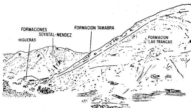
Figura 4.- Panorama del parautóctono en Higuerras. La barra calcárea de la Formación Tamabra forma la ceja y es de espesor muy delgado.
