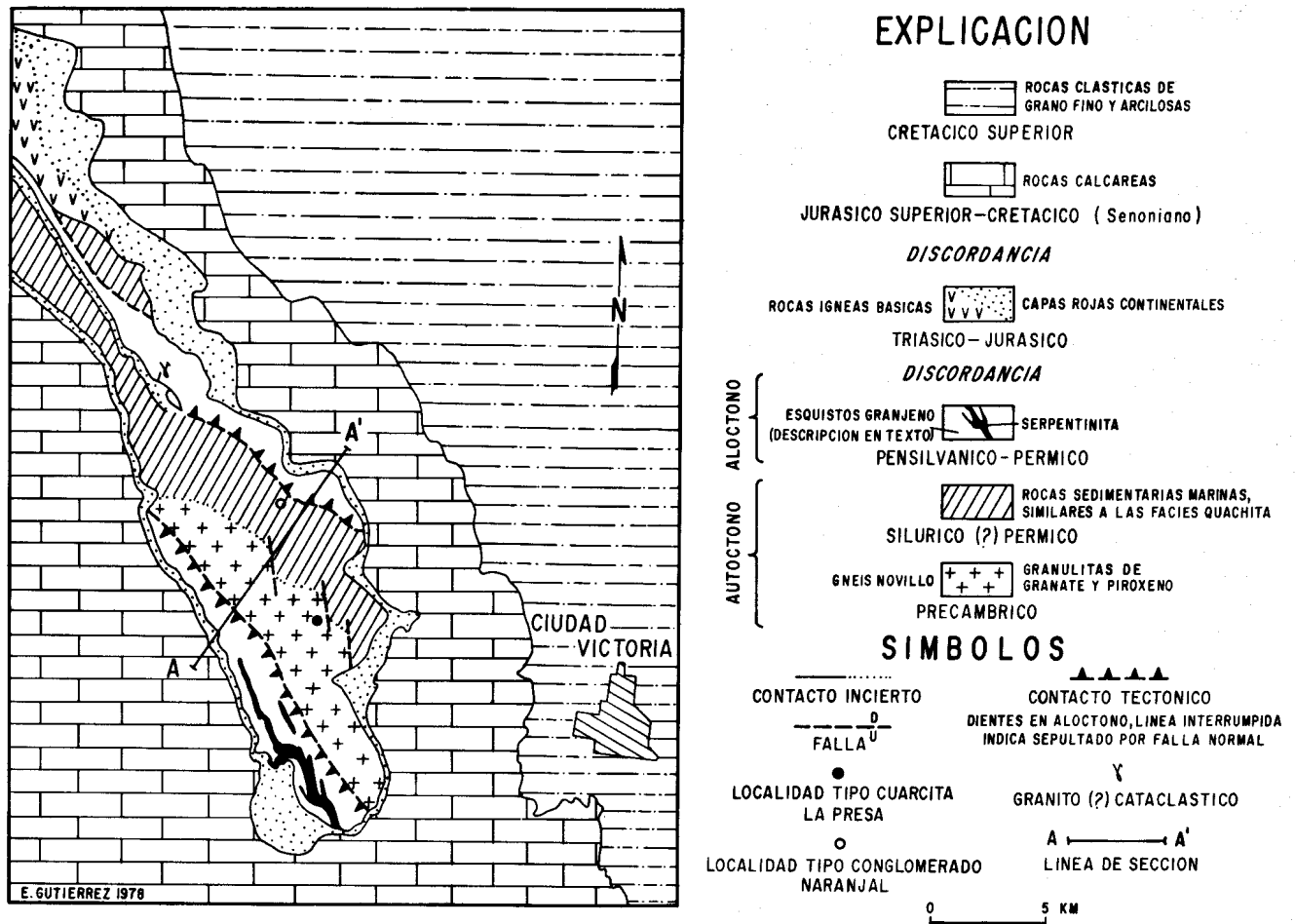
Figura 1.—Reinterpretación simplificada de la geología del Anticlinorio de Huizachal-Peregrina (parte norte). Modificada a partir de los datos de Carrillo-Bravo (1961), Fries y colegas (1962), Ramírez-Ramírez (1974) y de Cserna y colegas (1977).
