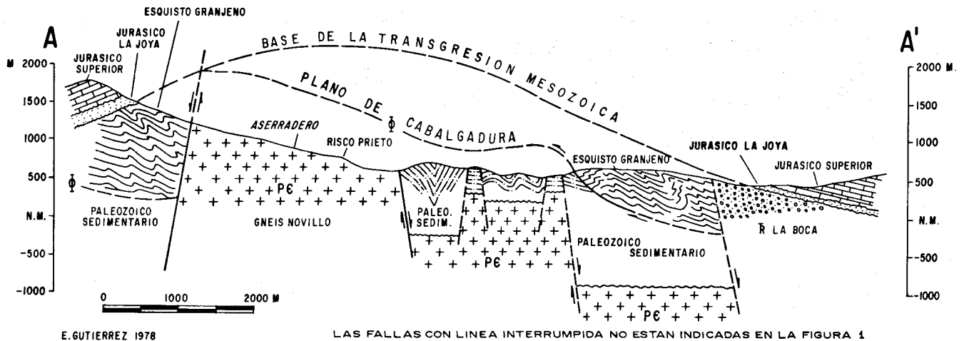
Figura 2.—Sección geológica interpretativa, basada en los datos de Carrillo-Bravo (1961), Ramírez-Ramírez (1974), y las observaciones hechas por Ramírez en 1976 y 1977. Topografía tomada de la sección C-C' de Ramírez-Ramírez ( op. cit. ).
