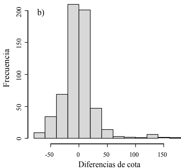
Figura 7. Histograma de frecuencia para (a) diferencias de anomalía de Bouguer (AB) y (b) diferencias de cota. Gráficos Q-Q para (c) diferencias de AB y (b) diferencias de cota. Nótese que las diferencias de AB presentan una distribución aparentemente normal y un buen ajuste a las rectas normales teóricas. Para las cotas hay valores extremos positivos que sesgan la distribución.
