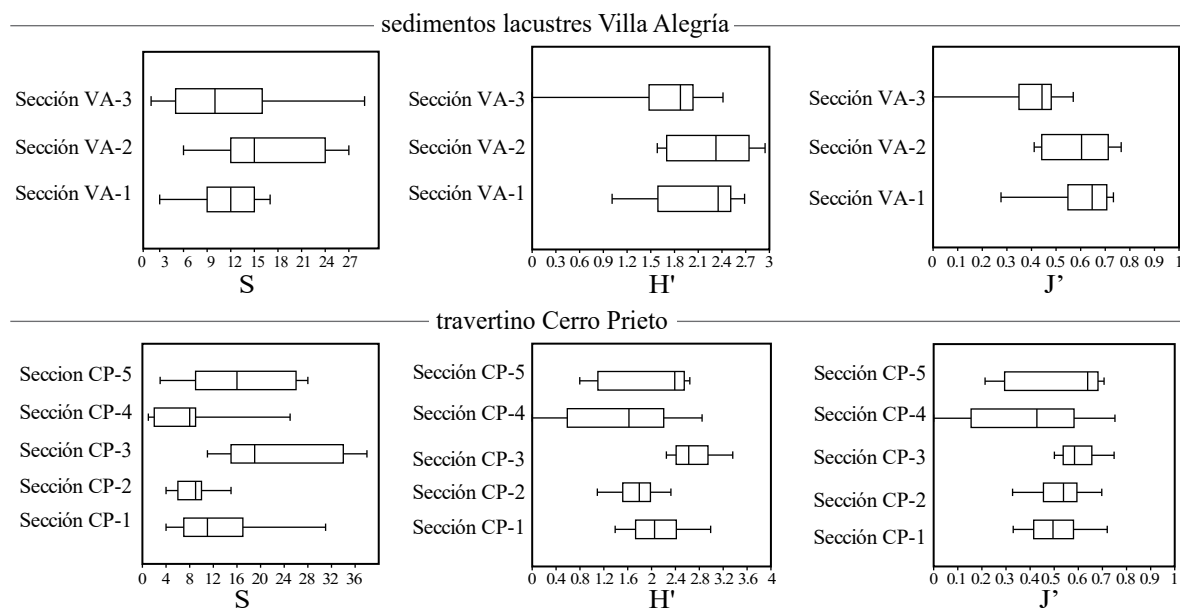
Figura 6. Rangos de riqueza de taxa (S), diversidad de Shannon-Wiener ( H' ) y equidad de Pielou ( J' ) obtenidos para las tres secciones de los sedimentos lacustres Villa Alegría y las cinco secciones del travertino Cerro Prieto.
