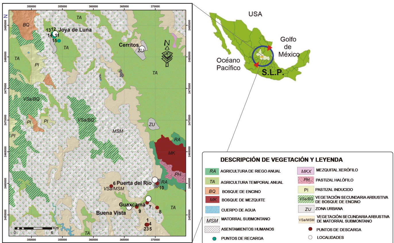
Figura 1. Localización del área de estudio en la porción central del Estado de San Luis Potosí (S.L.P.) y distribución de tipos de vegetación; se muestra la localización de los puntos de recarga y descarga de agua subterránea estudiados en la localidad Joya de la Luna y el área de Guaxcamá, respectivamente.
