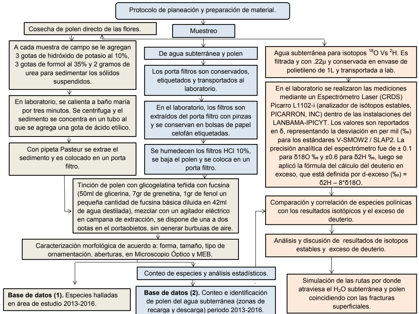
Figura 3. Diagrama de flujo de la metodología polínica ambiental (MEPAM).
