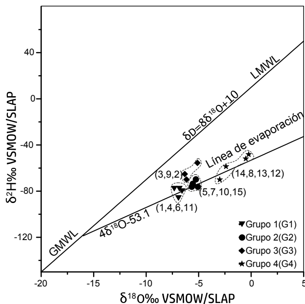
Figura 5. Relaciones isotópicas de las muestras de agua subterránea, normalizadas al patrón de Viena para la composición promedio del agua oceánica (VSMOW), y al patrón de precipitación ligera estándar del Antártico (SLAP). LMWL: Línea de agua meteórica local; GMWL: Línea de agua meteorológica global.
