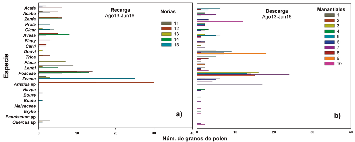
Figura 4. Especies identificadas vs. el número de granos de polen presentes en muestras de agua subterránea colectadas de (a) norias de la zona de recarga y (b) manantiales de la zona de descarga, en el periodo de agosto de 2013 a junio de 2016. Las abreviaturas de los nombres de las especies se definen en la Tabla 2 y la localización de los sitios de muestreo se presenta en las Figuras 1 y 2.
