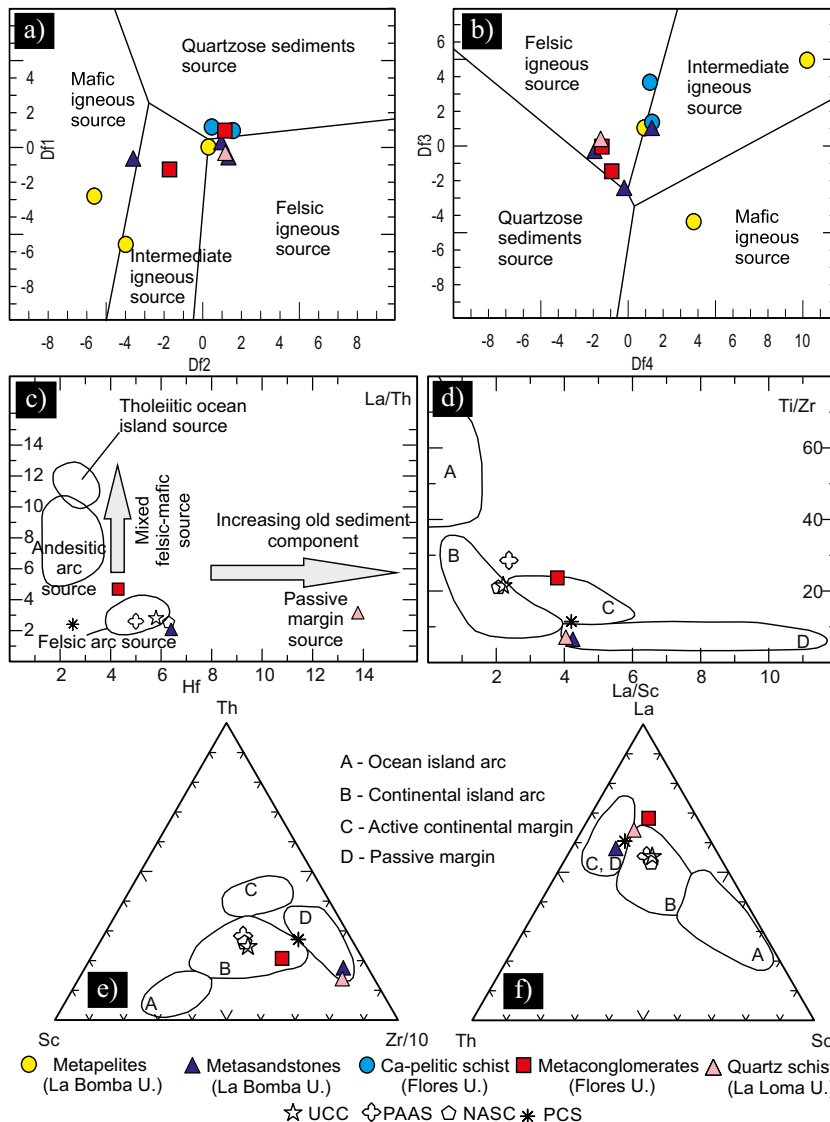
Figure 16. Source areas and tectonic setting diagrams. a) and b) Roser and Korsch, (1988). Discriminant function (Df) calculated as: Df1 = 56.500 TiO 2 /Al 2 O 3 - 10.879 Fe 2 O 3 /Al 2 O 3 + 30.875 MgO/Al 2 O 3 - 5.404 Na 2 O/Al 2 O 3 + 11.112 K 2 O/Al 2 O 3 - 3.89; Df2 = 30.638 TiO 2 /Al 2 O 3 - 12.541 Fe 2 O 3 /Al 2 O 3 + 7.329 MgO/Al 2 O 3 + 12.031 Na 2 O/Al 2 O 3 + 35.402 K 2 O/Al 2 O 3 - 6.382; Df3 = 0.445 TiO 2 + 0.070 Al 2 O 3 - 0.250 Fe 2 O 3 - 1.142 MgO + 0.438 CaO + 1.475 Na 2 O + 1.426 K 2 O - 6.861; Df4 = -1.773 TiO 2 + 0.607 Al 2 O 3 + 0.760 Fe 2 O 3 - 1.500 MgO + 0.616 CaO + 0.509 Na 2 O - 1.224 K 2 O - 9.090. In all discriminant functions Fe 2 O 3 represents total Fe content. c) Floyd and Leveridge (1987). d) - f) Bhatia and Crook (1986).
