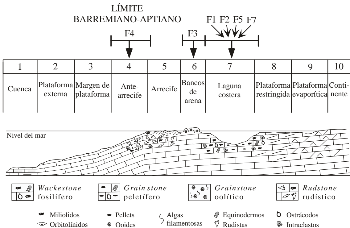
Figura 8. Perfil topográfico marino idealizado que muestra las Fajas de Facies Estándar sensu Wilson (1986) (1–10). Las flechas arriba indican el sitio de depósito de los paquetes de microfacies identificados en la sección estudiada (F1–F7), dentro de la reconstrucción paleoambiental. La transición Barremiano–Aptiano es coincidente con la unidad F4, localmente referida a un ambiente antearrecifal.
